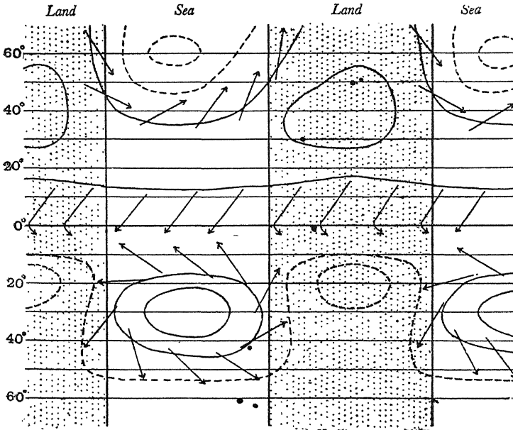
चित्र १३—जनवरी महीने में जमीन और समुद्र-सतह पर दाब के वितरण।
